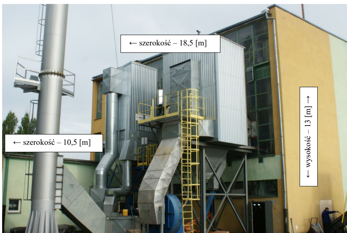
KOTŁOWNIA KR II – widok ściany kotłowni od strony filtrów.
